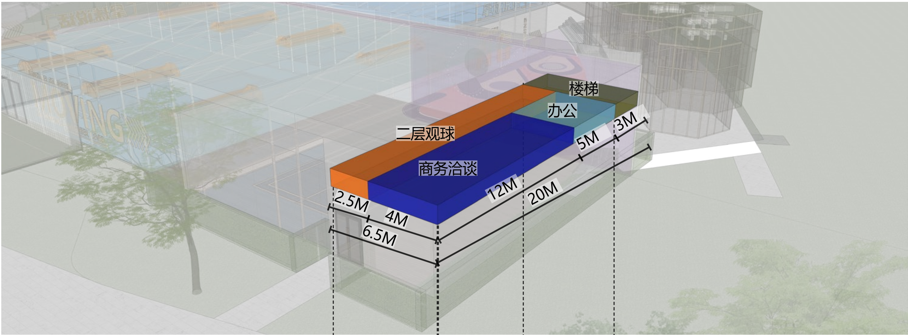
二层布局
